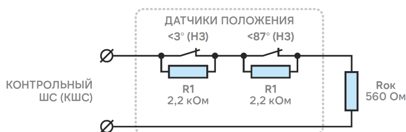
Рис.2. Схема подключения контрольного шлейфа сигнализации КШС. R_{ок} = 560 \text{ Ом} , R1 = 2,2 \text{ кОм} . Все резисторы \pm 5\% , 0,25 Вт. В дежурном режиме оба концевых выключателя в КШС должны быть замкнуты. При размыкании одного из контактов формируется «Сообщение 1» (например, «Клапан приоткрыт»), при двух разомкнутых контактах – «Сообщение 2» («Открыто»).
