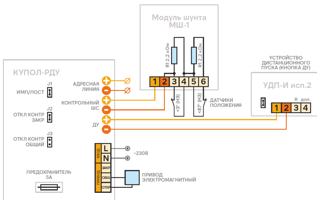
Рис.6. Схема подключения электромагнитного привода (нормально-выключенной нагрузки) с контролем наличия напряжения питания нагрузки.
