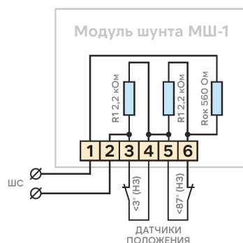
Рис.3. Модуль шунта МШ-1 для подключения к КШС.
