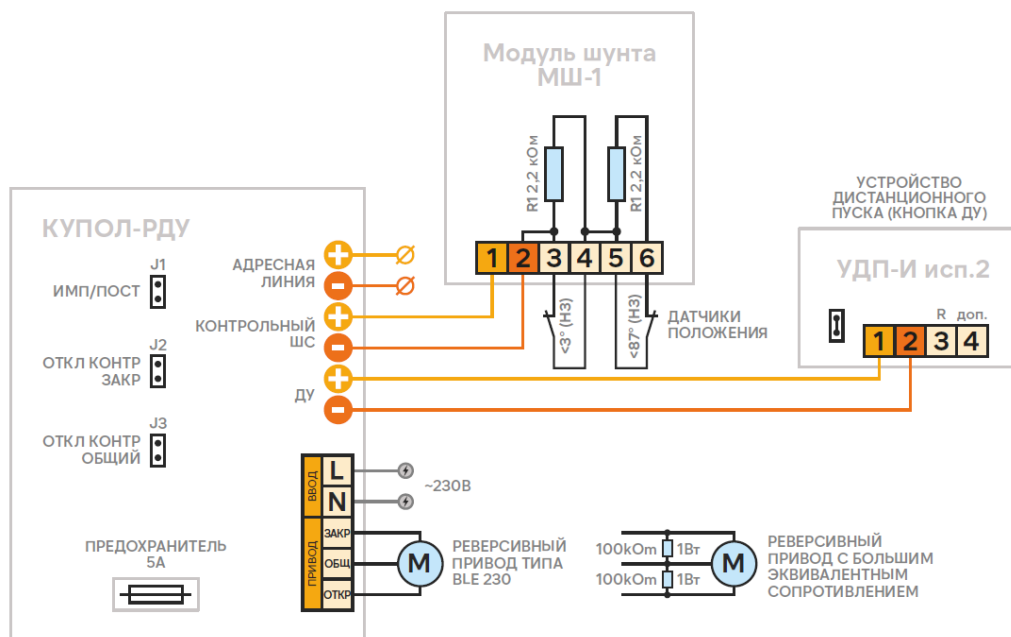
Рис.4. Схема подключения реверсивного привода типа «BLE 230» к КУПОЛ-РДУ. В зависимости от конструкции привода (например, привод производства Nanotek), при необходимости установить нагрузочные резисторы 100 кОм \pm 5\% , 1 Вт. Резисторы устанавливать в непосредственной близости от привода.
