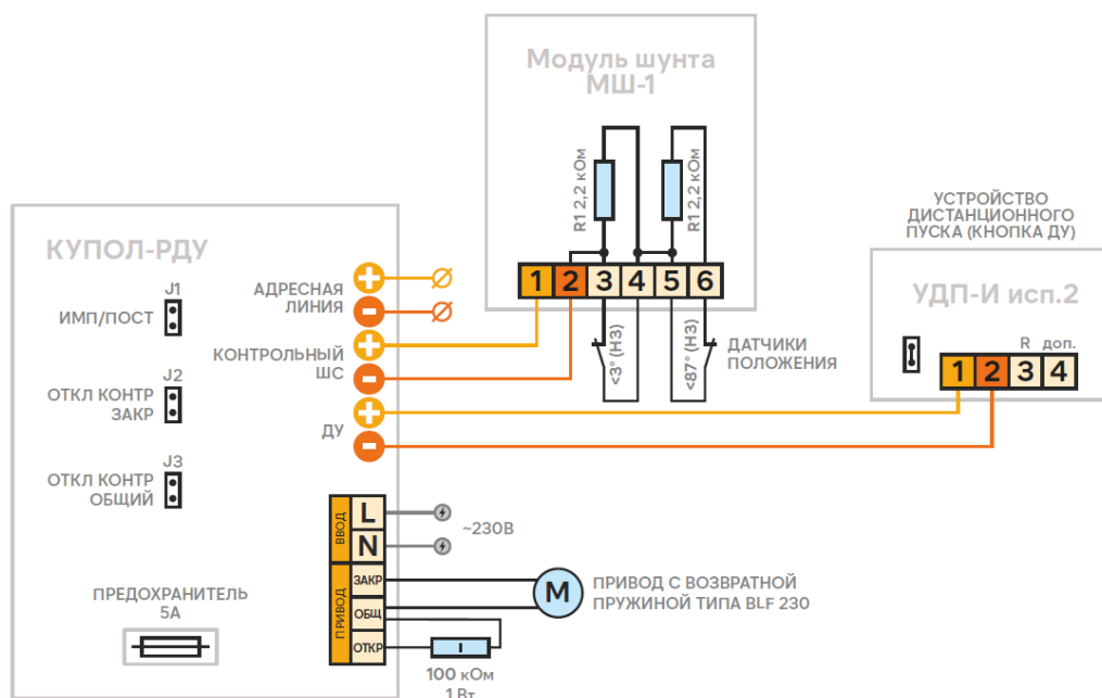
Рис.5. Схема подключения привода с возвратной пружиной типа «BLF 230» (нормально-включенной нагрузке) с контролем наличия напряжения питания нагрузки.
